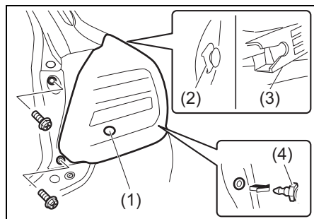
(1) 方向指示器／非常点滅表示灯 (後面、Aタイプ)
